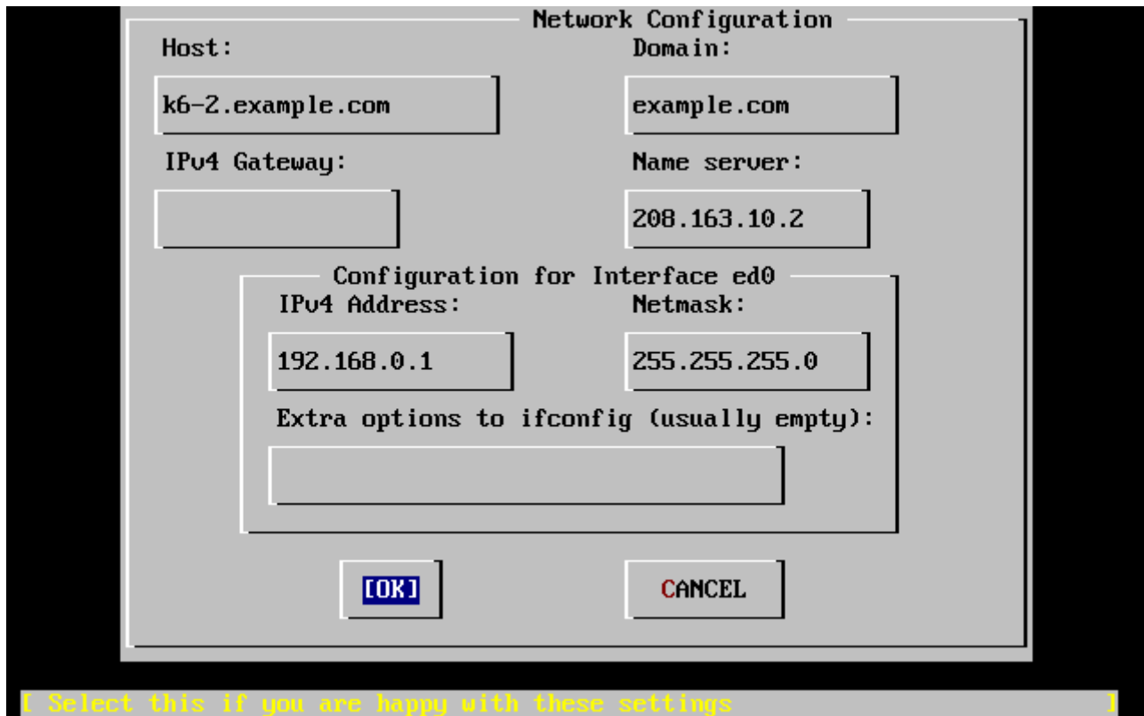
Рисунок 28. Настройка сети для ed0
