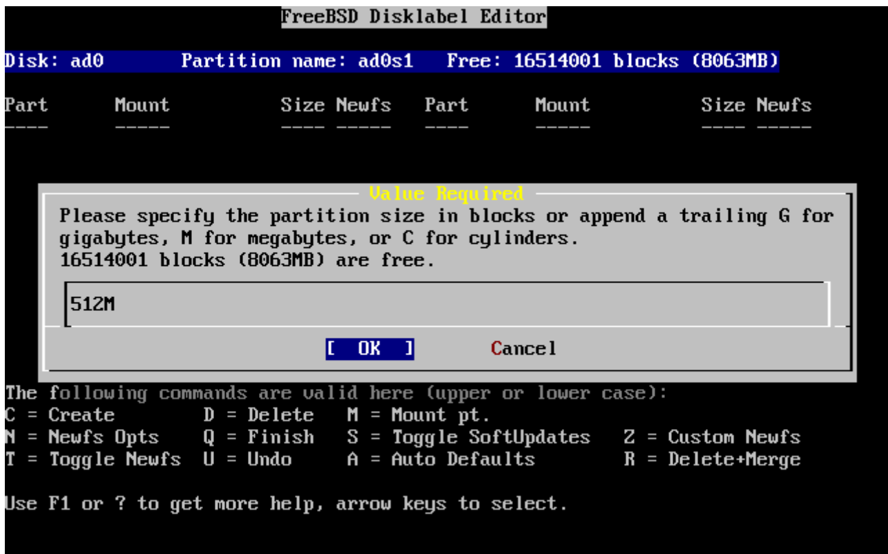
Рисунок 20. Редактирование размера корневого раздела
