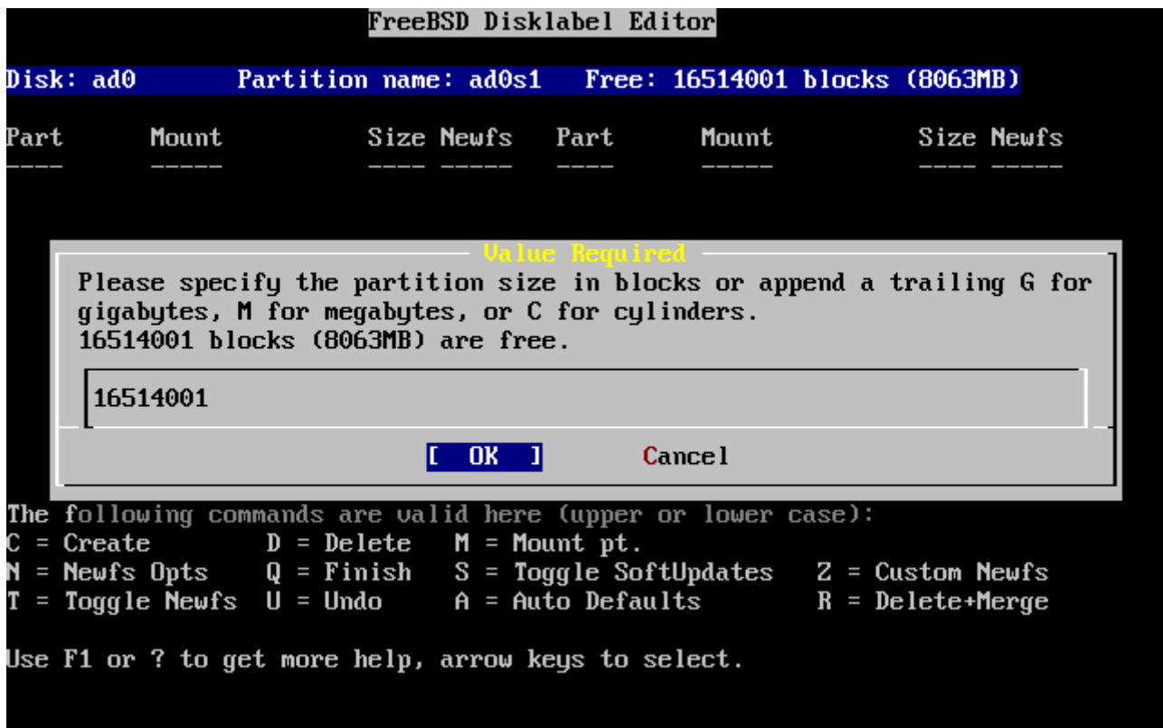
Рисунок 19. Свободное место для корневого раздела
